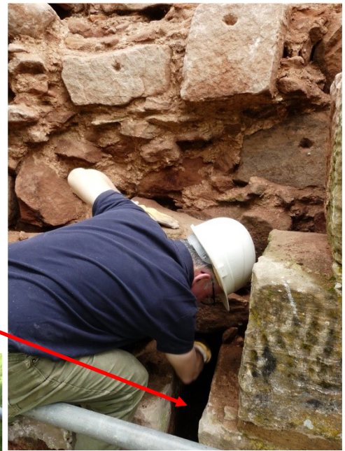
Canal d'évacuation d'eau traversant le rempart.
